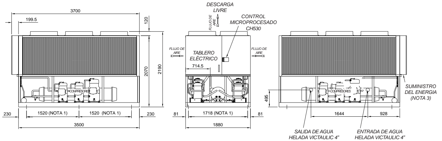
Fig. 21 - Dimensiones de la Unidad CGAD 070
