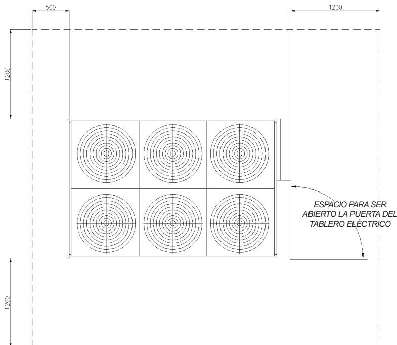
Fig. 20 - Espacios para mantenimiento y circulación de aire.
