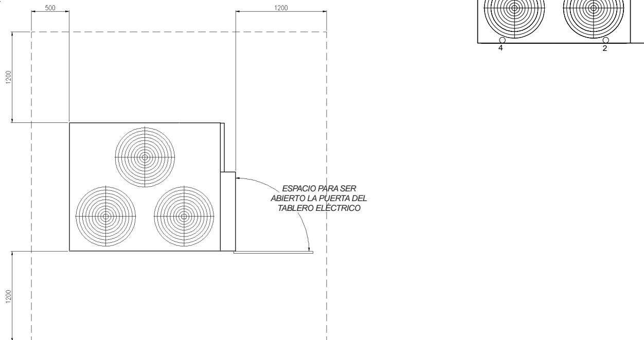
Fig. 14 - Espacios para mantenimiento y circulación de aire.
