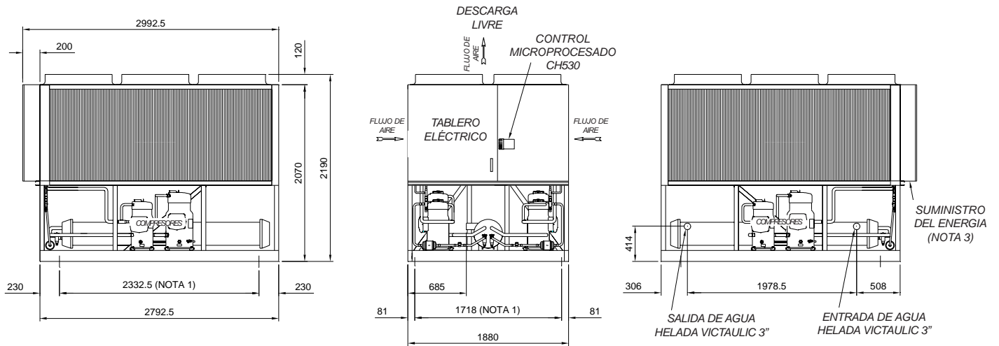
Fig. 17 - Dimensiones de la Unidad CGAD 050
