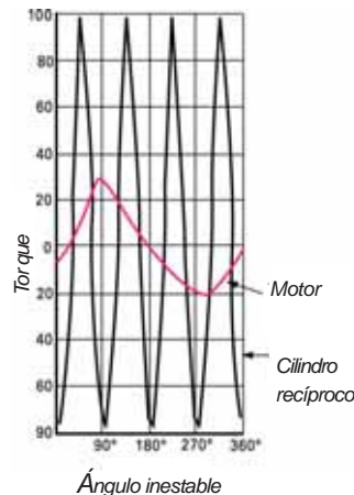
Fig. 39 - Comparativo Scroll x Recíproco
